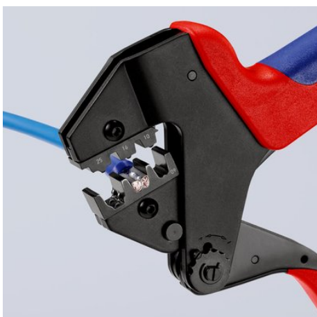
97 43 200 s lisovacím nástavcem 97 49 06 pro izolovaná kabelová oka, konektory a dvojité spojky
