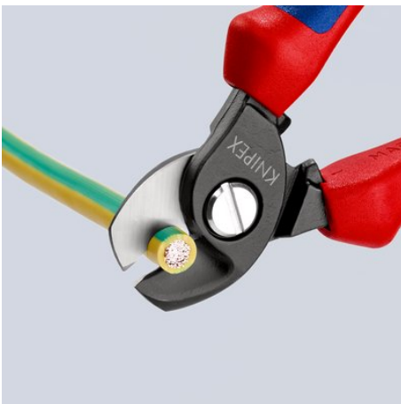
Prestřížení kabelu kleštěmi na kabely: lehký, čistý řez bez deformace kabelu
