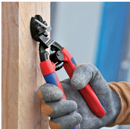
hlava nahnutá v úhlu 20° s jednostrannou klopou a se zařízutím strany pro rovné řezání; s volným prostorem pro uchopení
